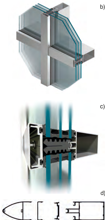
Rys. 4. Szklano-metalowa fasada słupowo-ryglowa a) widok przykładowej fasady z wnętrza pomieszczenia, b) detał konstrukcyjny, c) wizualizacja połączenia szyby termoizolacyjnej i kształtownika nośnego z elementem mocującym zestaw szybowy, d) przykłady przekrojów poprzecznych aluminiowych profili składowych systemu fasadowego (b/c/d – Aluprof – MB-SR50N).
