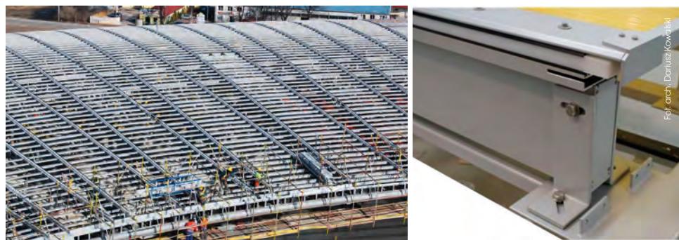
Rys. 5. Przykład zastosowania aluminium na konstrukcję wsporczą pod poszycie zadaszenia a) fragment konstrukcji nośnej zadaszenia stadionu z zamontowanym rusztem nośnym z wyciskanych profili aluminiowych i układem promieniowych rynien wykonanych z blachy aluminiowej, b) detał połączenia wraz aluminiowym okuciem z aluminium poszycia poliwęglanowego
