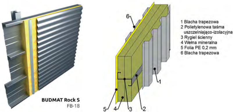
Rys. 12. Ściana wentylowana: a) z kaset ściennych ocieplana wełną mineralną i zewnętrzną warstwą osłonową z płyty falistej (Budmat), b) z wełny mineralnej umieszczonej pomiędzy ryglami i zewnętrznymi warstwami z blachy trapezowej (Commercecon)
