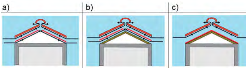
Rys. 13. Działanie wentylacji dachu spadzistego: a) dach tradycyjny z wentylowanym, nieużywanym poddaszem, b) dach z poddaszem ocieplonym z rozpiętą folią wstępnego krycia i dwoma strefami wentylacyjnymi, c) współczesny dach ocieplony z jedną strefą wentylacyjną (www.dachy.info.pl)
