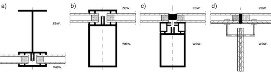
Rys. 5. Proces modyfikacji konstrukcji ściany słupowo-ryglowej a) Detal ściany słupowo-ryglowej starego typu. Konstrukcja ściany usytuowana na zewnątrz budynku, po jej stronie zimnej. Oszklenie ściany montowane od wewnątrz budynku b) Detal ściany słupowo-ryglowej nowej generacji. Konstrukcja ściany usytuowana na wewnętrznej stronie przegrody, po jej stronie ciepłej. Oszklenie ściany montowane od zewnętrznej strony budynku c) Detal ściany słupowo-ryglowej z oszkleniem strukturalnym. Konstrukcja ściany usytuowana po wewnętrznej stronie przegrody, po jej cieplej stronie. Oszklenie ściany montowane od strony zewnętrznej budynku d) Detal ściany osłonowej z punktowym (mechanicznym) mocowaniem oszklenia (nowej generacji). Konstrukcja przegrody usytuowana po jej stronie wewnętrznej (żebro szklane)
