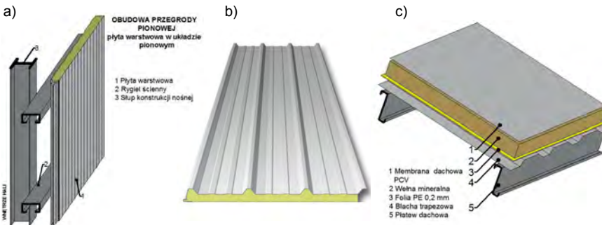
Rys. 11. Przykładowe przegrody warstwowe niewentylowane: a) ściany z płyty warstwowej, pokrycia dachowe: b) z płyty warstwowej; c) na blasze trapezowej (Commercecon, Florian Centrum SA)
