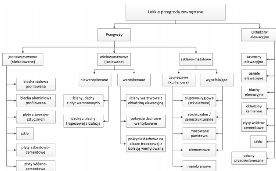
Rys. 1. Klasyfikacja lekkich przegród zewnętrznych (autorzy)
