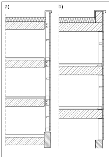
Rys. 3. Rodzaje fasad: a) ściana typu zawieszona (kurtynowa), b) ściana wypełniająca
