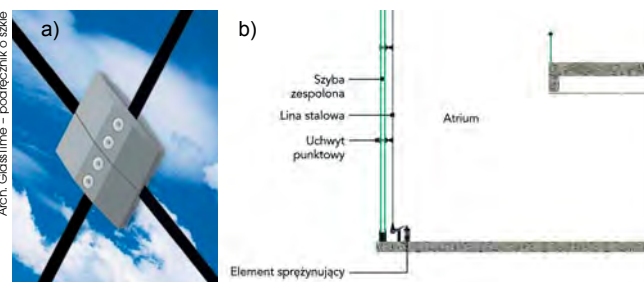
Rys. 8. Przykłady rozwiązań konstrukcyjnych ścian z oszkleniem mocowanym punktowo
