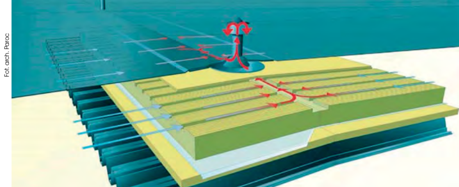
Rys. 15. System wentylowanej izolacji dachów płaskich PAROC® Air
