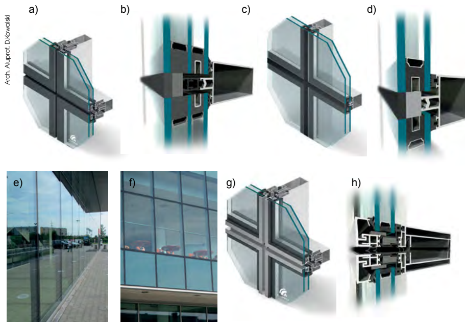
Rys. 6. Przykłady rozwiązań konstrukcyjnych ścian z oszkleniem strukturalnym
