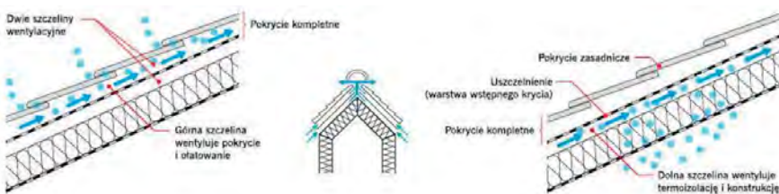
Rys. 14. Zasada działania wentylacji: w dachu z dwiema szczelinami (www.infoarchitekta.pl)
