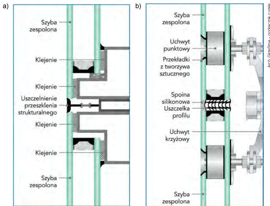
Rys. 7. Techniki mocowania oszklenia: a) szklenie strukturalne, b) mocowanie punktowe
