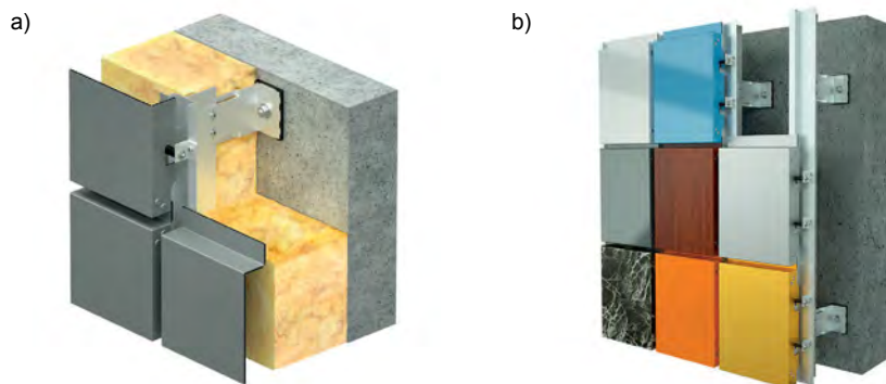
Rys. 16. Konstrukcja fasady wentylowanej z okładziną metalową: a) izolowanej, b) bez warstwy izolacyjnej (Aluprof, system EXTRABOND)
