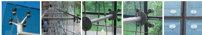
Rys. 8. Przykłady rozwiązań konstrukcyjnych ścian z oszkleniem mocowanym punktowo
