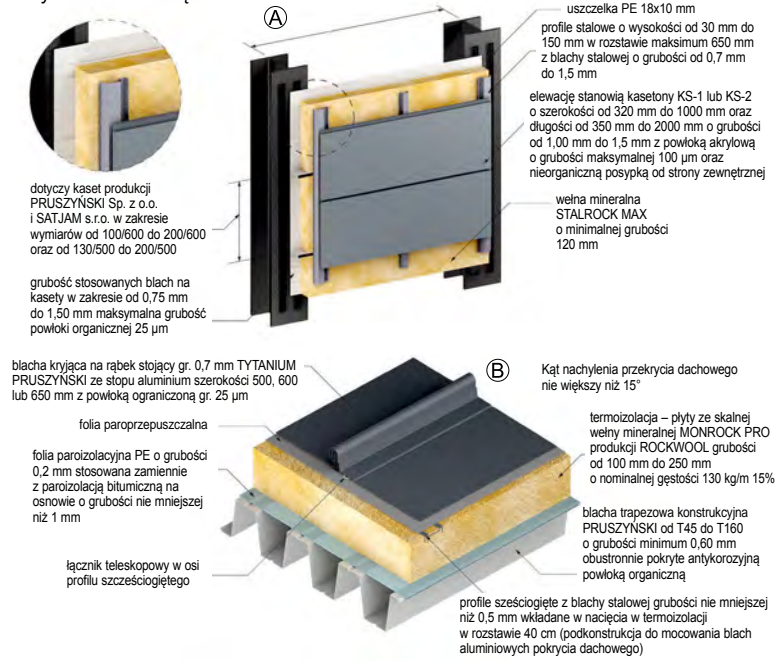
W nadbudowie można wykorzystać system lekkich ścian osłonowych opartych na kasetach ściennych wypełnionych wełną mineralną (A), oraz do konstrukcji dachu nadbudowy - lekką obudowę opartą na blasze trapezowej (B).
