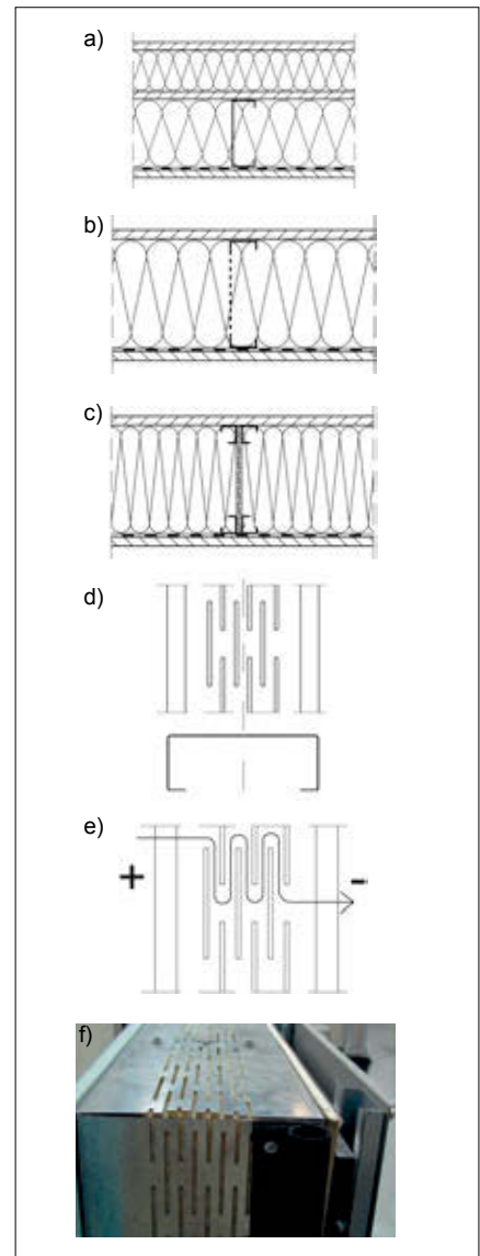
Rys. 12. Metody eliminacji mostków cieplnych w lekkich przegrodach z zastosowanymi elementami metalowymi nośnymi (dystansowymi) [4]: a) dodatkowa warstwa izolacyjna, b) zastosowanie kształownika z perforowanym środkiem, c) zastosowanie na konstrukcję środka przekładki z innego materiału, np. sklejki, d) przykładowy ceownik z perforowanym środkiem – system TERMO, e) wydłużona ścieżka przepływu ciepła przez metalowy kształownik spowodowana wykonaniem odpowiednich perforacji, f) przykład konstrukcji ściany z zastosowaniem kształownika perforowanego – system TERMO
