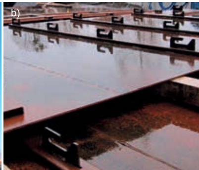
Rys. 9. Przykład zastosowania okładziny ze stali typu Cor-Ten, o podwyższonej odporności na warunki atmosferyczne, na budynku ECS w Gdańsku: a) fragment elewacji budynku, b) składowana blacha elewacyjna z widocznymi zawieszami
